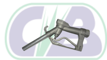
Bico descarga alumínio 19mm e 25mm - CB TOOLS
